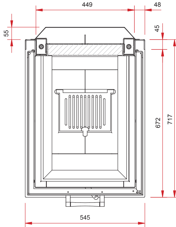
Draufsicht M 1:10
