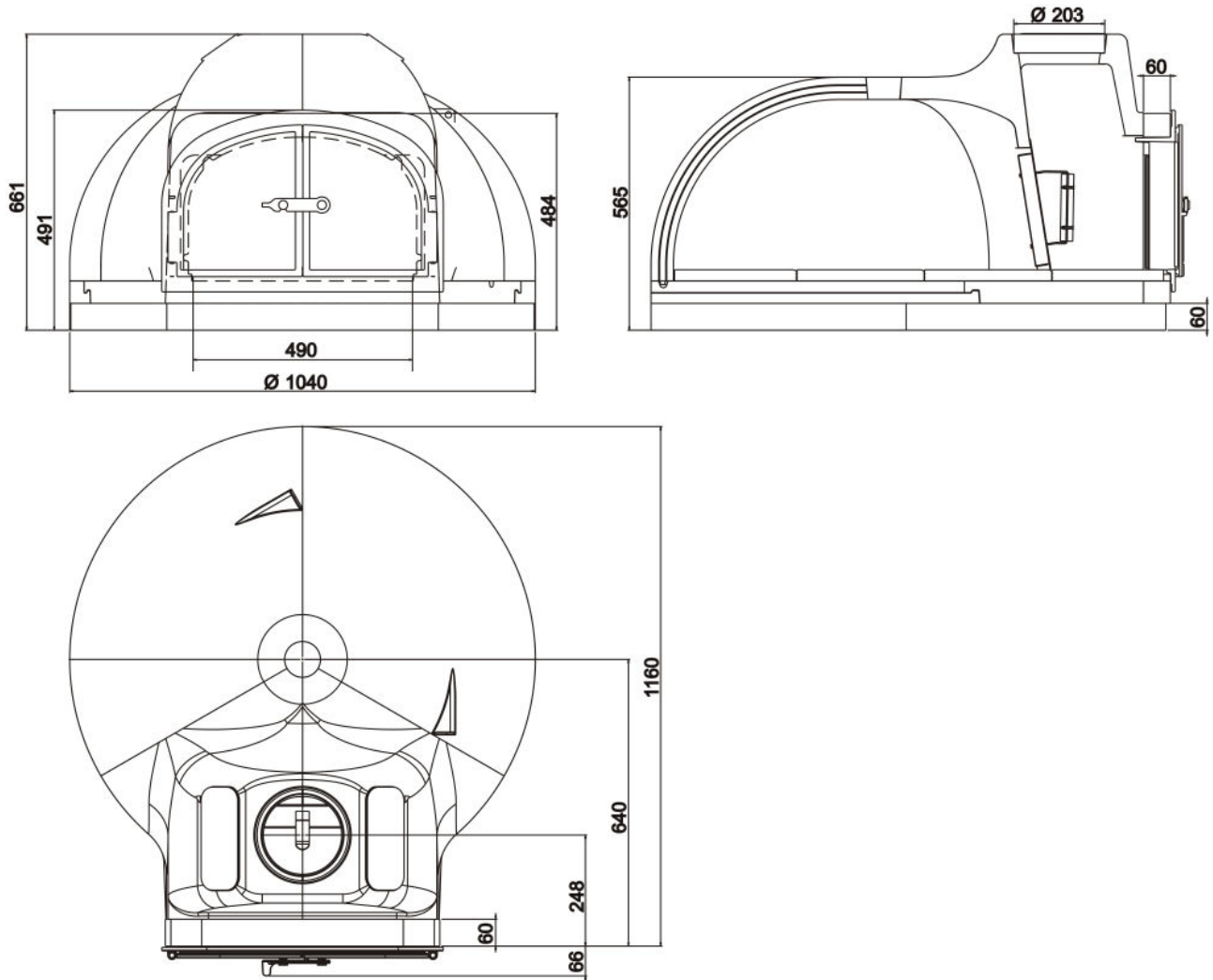
Abb.2: Feuer Iglu 950 mit Gußtür
