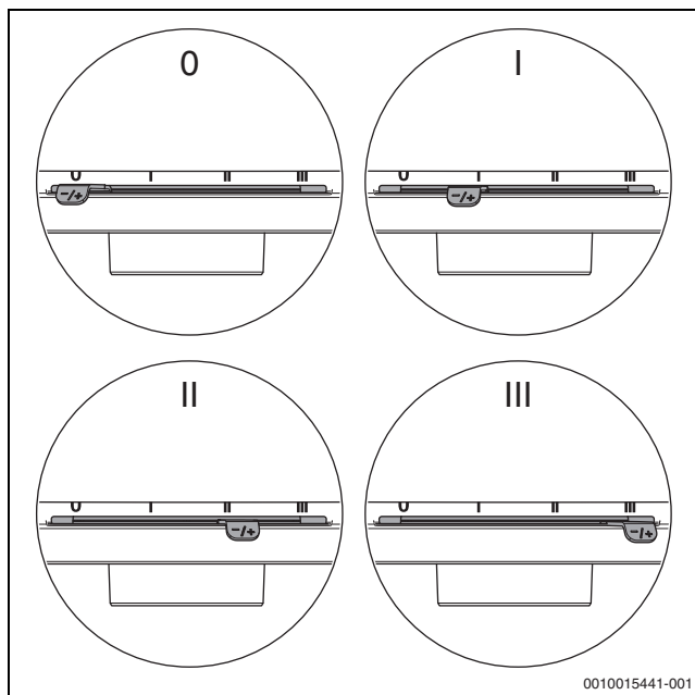
Bild 8 Verbrennungsluftschieber regulieren
