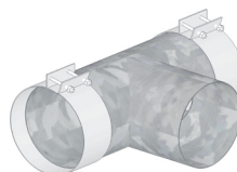
1x T-Stück 150mm Rohr mit 2 Schellen
