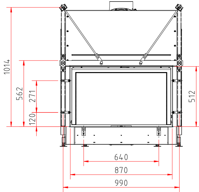
Frontansicht M 1:20
