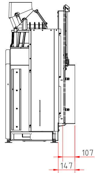
Seitenansicht M 1:20
