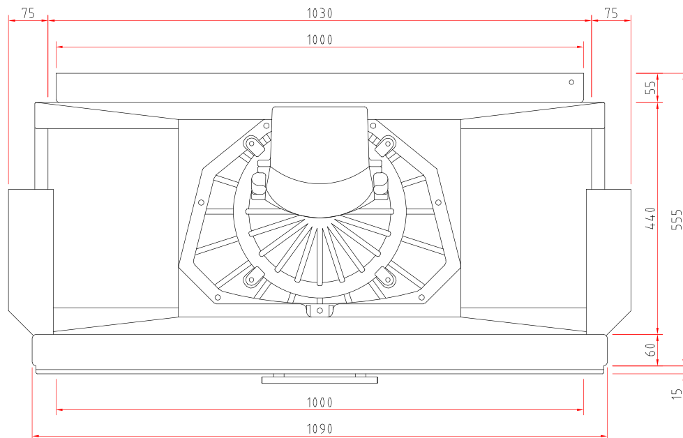
Draufsicht M 1:10
