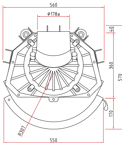
Draufsicht M 1:10
