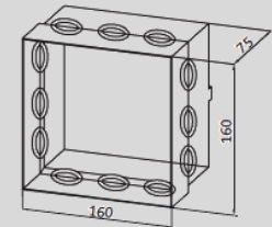
Der Unterputzkasten für die Ofensteuerung wird in einem kalten Wandbereich auf Sichthöhe montiert.
