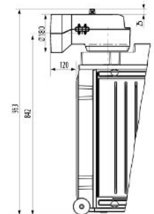
DIAMANT H13 mit waagrechttem Heizgasstutzen Ø 180mm (Zubehör)
