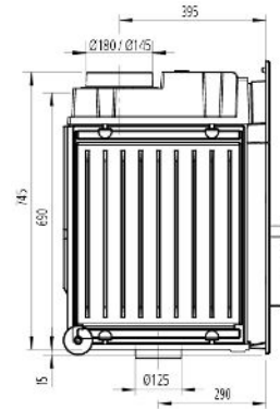
DIAMANT H10, Seitenansicht
