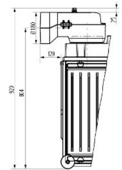
DIAMANT H10 mit waagrechttem Heizgasstutzen Ø 180mm (Zubehör)
