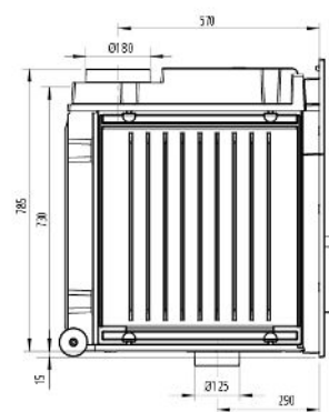
DIAMANT H13, Seitenansicht
