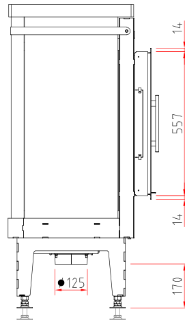
Seitenansicht M 1:20
