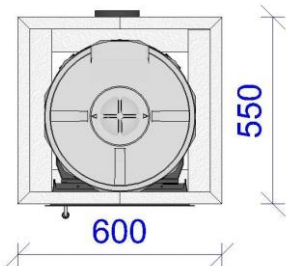
Draufsicht
