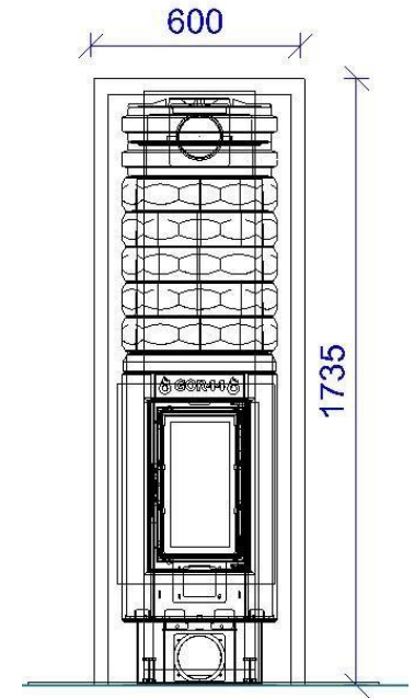
Seitendarstellung
