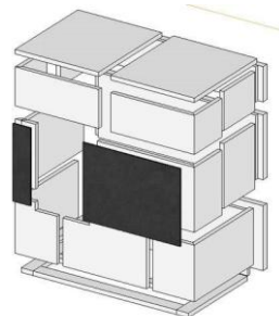
Explosionszeichnung
