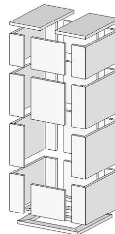
Explosionszeichnung
