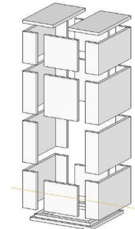
Explosionszeichnung
